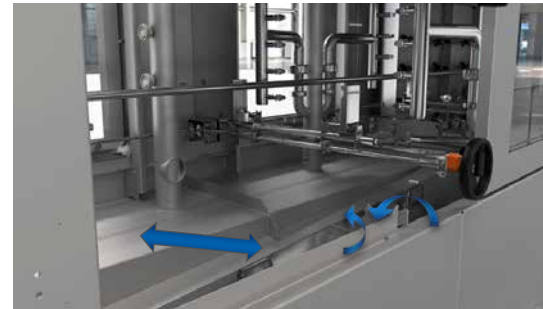
La anchura del rociado a alta presión se puede ajustar de forma continua.
