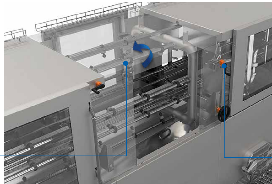
Tubos rociadores de cierre rápido para fácil montaje y desmontaje
