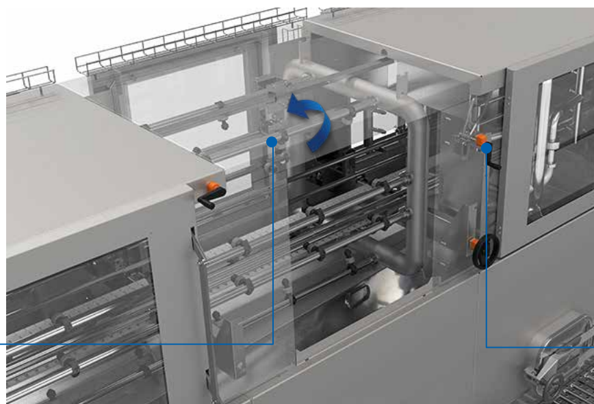
喷管的快速封盖实现简易的安装和拆卸
