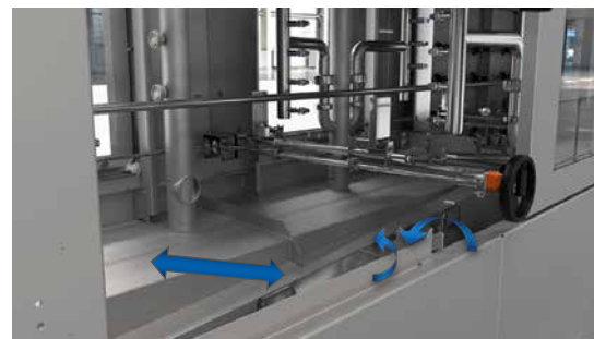
高压喷淋装置的宽度可无极调节。
